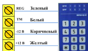
Рис. 8.4. Схема подключения кодовой панели Мираж-КД
