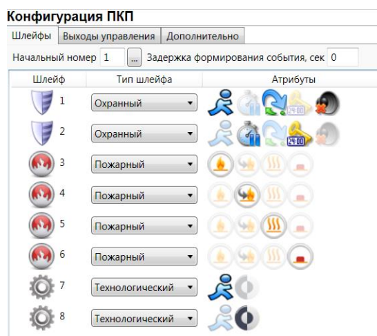
Рис. 5.8. Вкладка Шлейфы
