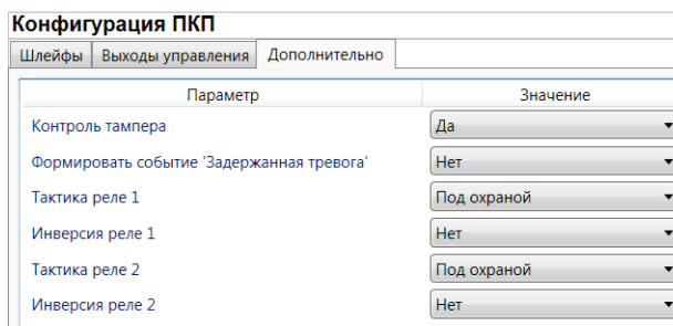
Рис. 5.11. Вкладка Дополнительно
