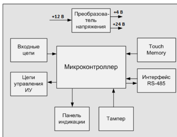
Рис. 3.1. Функциональная схема
