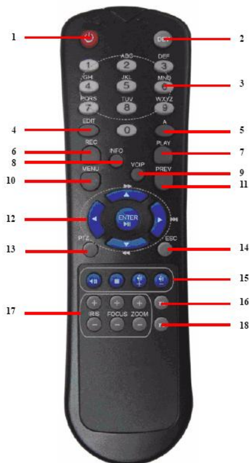
Рис 1.1 Пульт дистанционного управления
