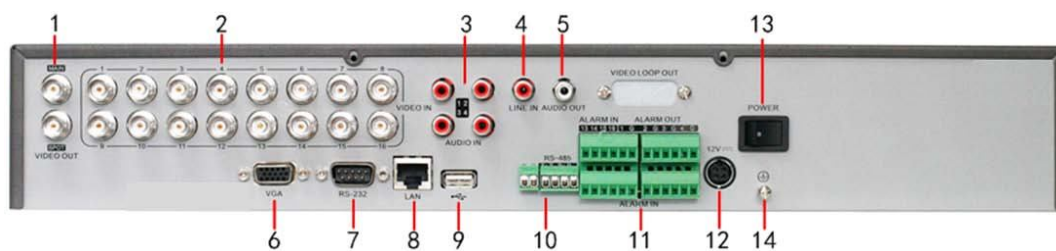
Figure 17. Задняя панель DSR-1605-h
