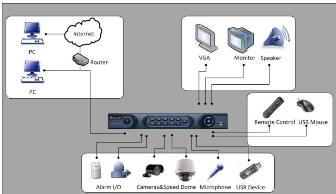
Рис.6. Подключение устройства
