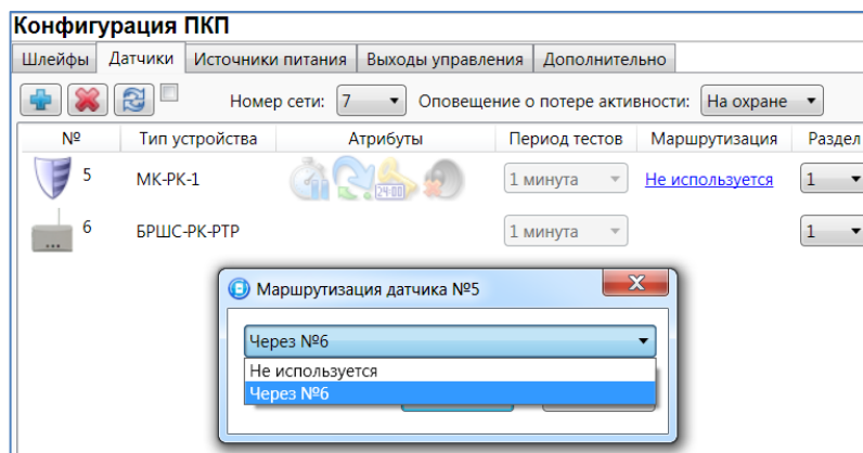
Рис. 5.9. Настройка маршрутизации радиопередатчиков
