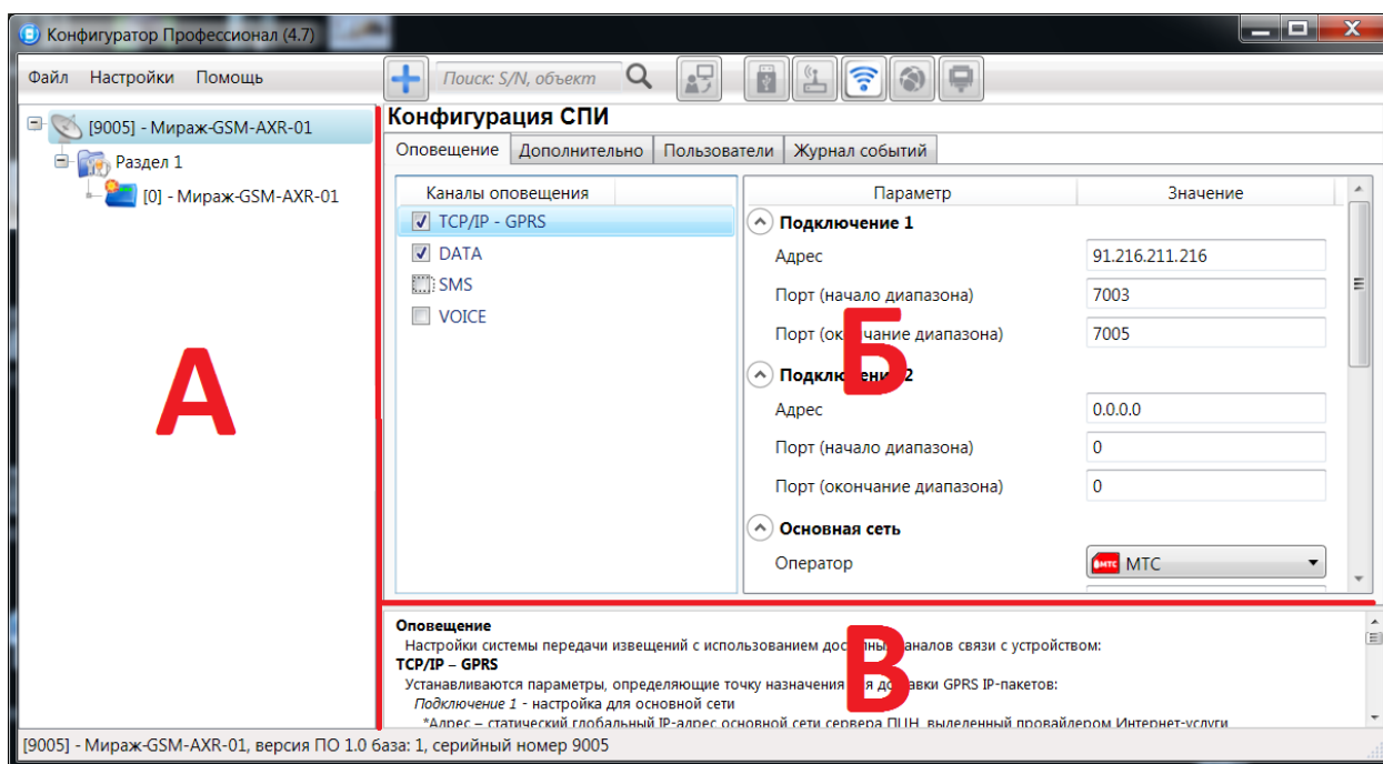
Рис.6.1. Структура основного окна программы Конфигуратор Профессионал 4.7 (А — дерево устройств, Б — область параметров, В — область подсказок)
