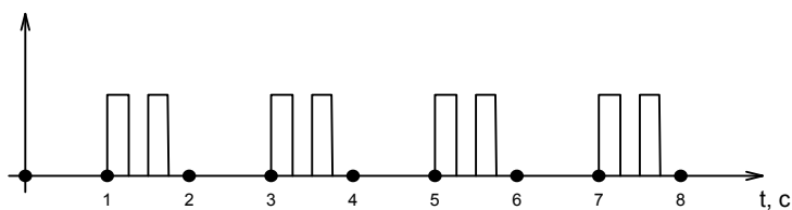
Рис. 3.7. Индикация наличия соединения по каналу TCP/IP GPRS
