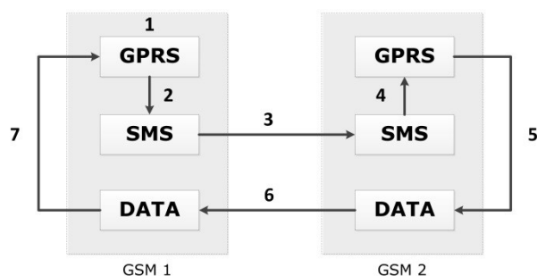
Рис. 4.2. Алгоритм оповещения о тревожных событиях при поддержании TCP/IP-соединения (отправке тестовых TCP/IP-пакетов)
