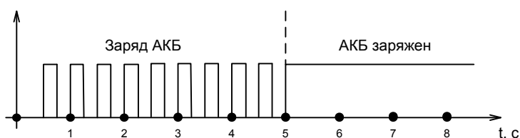
Рис. 3.8. Индикация зарядки АКБ
