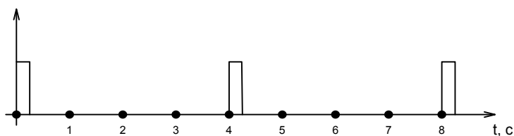
Рис. 3.4. Индикация недоступности каналов доставки извещений
