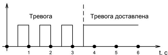
Рис. 3.3 Индикация режима тревоги
