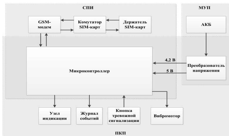
Рис. 3.1. Функциональная схема
