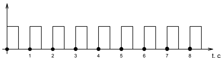
Рис. 3.9. Индикация режима конфигурирования
